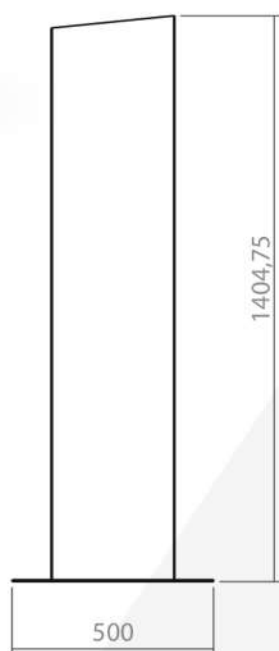
Vista Lateral
